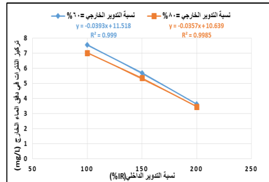
الشكل (6) العلاقة بين تركيز النترات (NO 3 -N) في دفق الماء الخارج عند نسبتي التدوير الداخلي (IR%) والخارجي (RAS%)
