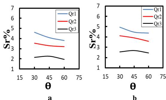
شكل رقم (11) يوضح العلاقة بين زاوية التفرع ونسبة الرسوبيات الداخلة الى قناة المأخذ عند Q_m = 12 \text{ L/s} , Q_{r1} = 7 \text{ L/s} (a) Q_{r2} = 2.22 \text{ g/s} (b) Q_{r3} = 1.8 \text{ g/s}
