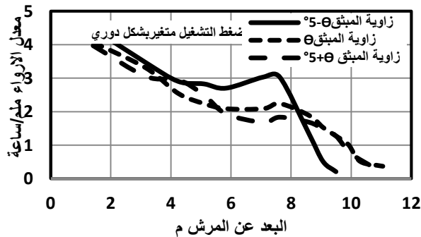
الشكل (7): مقارنة بين نمط توزيع الماء على امتداد الشعاع الذي يمثل نصف قطر دائرة الإبتلال للمرشة لقيم مختلفة لزواية المبتق 5+\theta ، \theta ، 5-\theta وذلك عند ضغط تشغيل ثابت و ضغط تشغيل متغير بشكل دوري لرأس المرش GESU
