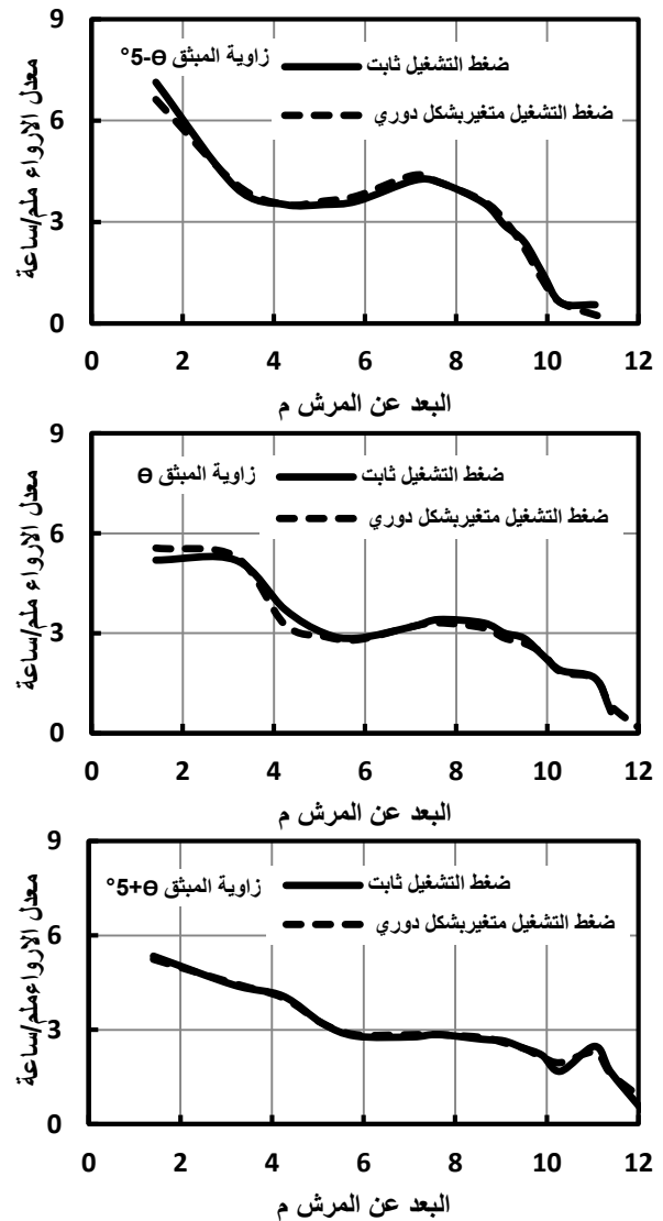
الشكل (9): مقارنة بين نمط توزيع الماء على امتداد الشعاع الذي يمثل نصف قطر دائرة الابتلال للمرشة عند ضغط تشغيل ثابت وضغط تشغيل متغير بشكل دوري لحالات مختلفة لزواية المبيتق وذلك لرأس المرش Rain bird.
