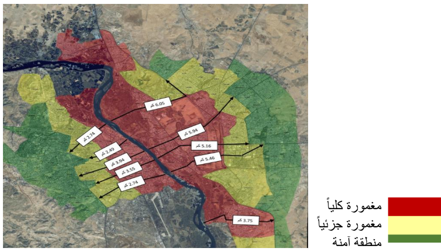
الشكل (8): خريطة الاحياء المغمورة كلياً وجزئياً والامنة لمدينة الموصل وبُعد الأماكن الامنة عن حافة النهر لسيناريو الانهيار الافتراضي اللحظي لسد الموصل عند منسوب خزن (335) متراً.
