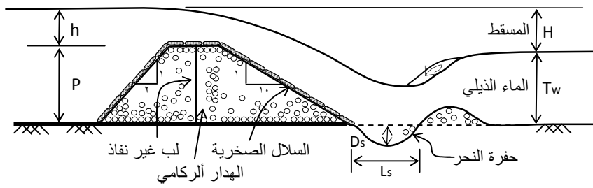
المقطع (B-B): مخطط توضيحي للسد ألركامي والنحر أثناء التشغيل
