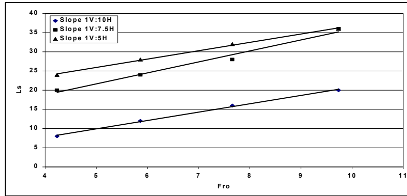
الشكل (٦): العلاقة بين طول حفرة النحر و Fro لـ ( 1.11 = dm )
