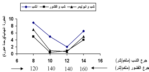
شكل 4: يمثل العكورة النهائية لمياه خام بعكورة ابتدائية (40) وحدة عكورة بعد معاملتها باستخدام الشب لوحده والشب مع قشور الجوز والشب مع (0.05) ملغم /لتر بولي الكتروليت.
