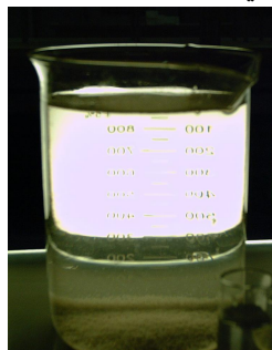
الشكل 11: صور توضح خصائص الحمأة المتكونة باستخدام أ- الشب لوحده ب- الشب مع البولي الكتروليت ج- الشب مع قشور الجوز
