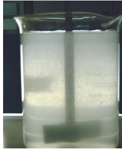
الشكل (9): صور توضح تكون اللبادات بعد مرور 5 دقائق من المزج البطيء باستخدام أ- الشب لوحده ب- الشب مع البولي الكتروليت ج- الشب مع قشور الجوز
