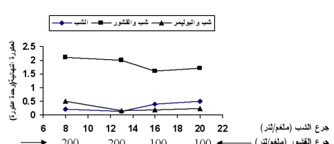
شكل 5: يمثل العكورة النهائية لمياه خام بعكورة ابتدائية (50) وحدة عكورة بعد معاملتها باستخدام الشب لوحده والشب مع قشور الجوز والشب مع (0.05) ملغم /لتر بولي الكتروليت.
