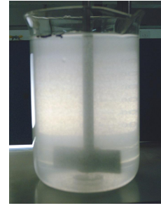
الشكل (9): صور توضح تكون اللبادات بعد مرور 5 دقائق من المزج البطيء باستخدام أ- الشب لوحده ب- الشب مع البولي الكتروليت ج- الشب مع قشور الجوز
