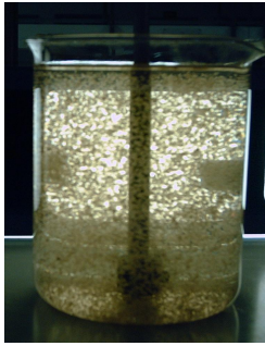
الشكل (10): صور توضح تكون اللبادات في نهاية المزج البطيء باستخدام أ- الشب لوحده ب- الشب مع البولي الكتروليت ج- الشب مع قشور الجوز
