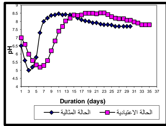
الشكل (7) تغاير الرقم الهيدروجيني لمزيج النفايات داخل البراميل خلال فترة تكوين الدبال في موسم الشتاء
