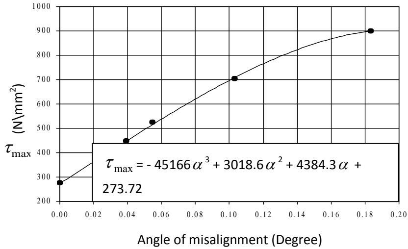
الشكل (9): تزايد أكبر قيمة متولدة لإجهاد \tau_{max} زاوية عدم المحاذاة
