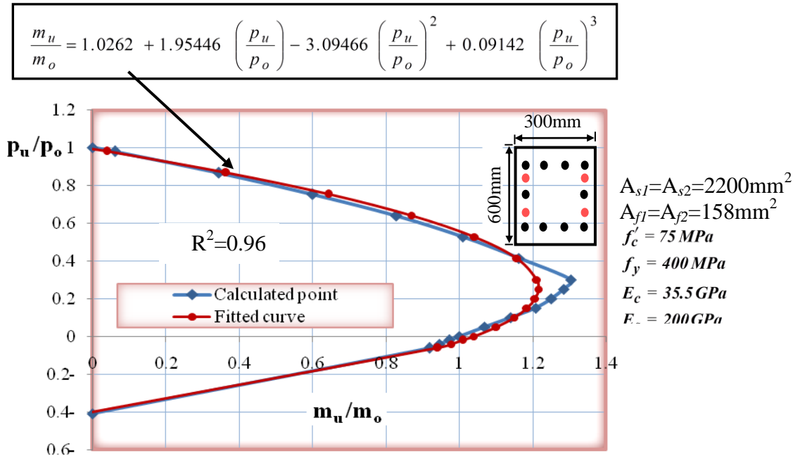
الشكل (9): يوضح منحنى التداخل الحقيقي والتوافق للقوة المحورية والعزم
