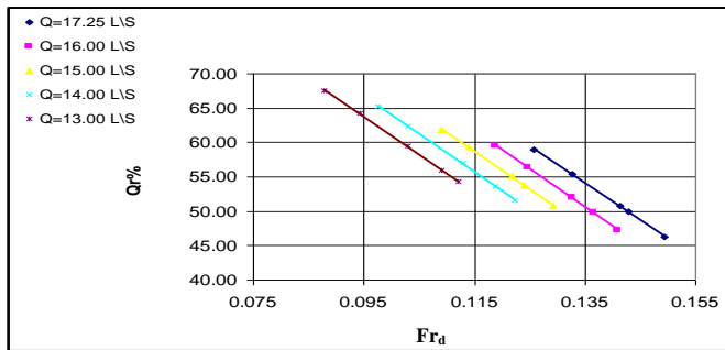
الشكل (5): العلاقة بين نسبة التصريف المتفرع ورقم فرود في مؤخر
