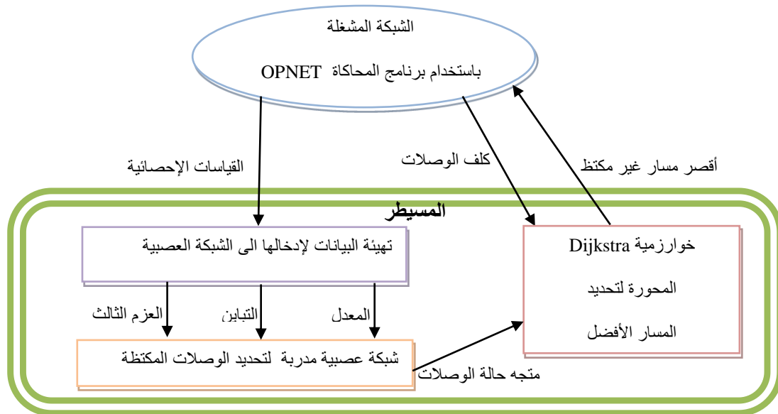
الشكل (2): الإطار العام لعمل الخوارزمية المقترحة
