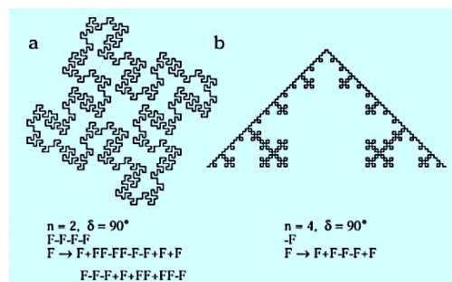
الشكل(13) يوضح توليد (منحنيات Koch) باستخدام احكام التفسير في نظام لندنماير.
