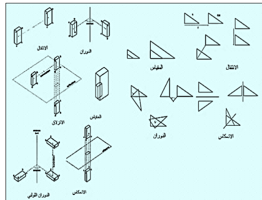
الشكل (14 أ) تحولات شكلية ثنائية الابعاد
