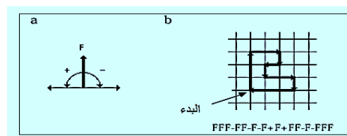
الشكل(12)احكام التفسير في نظام لندنماير. (Prusinkiewicz & Lindenmayer, 1990, p.7)
